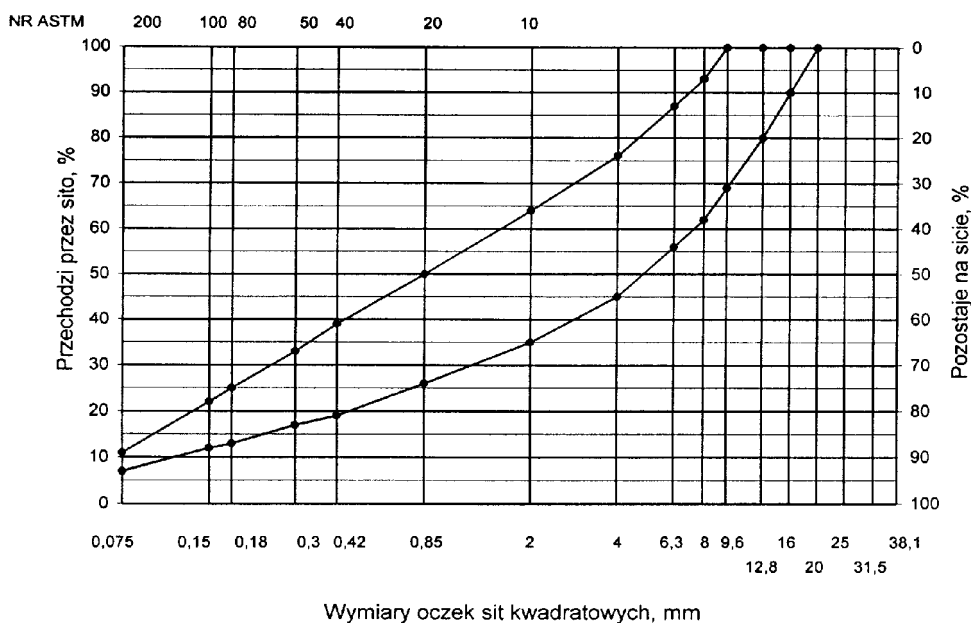
Rys. 1. Krzywe graniczne uziarnienia mieszanki mineralnej BA od 0 do 16mm, od 0 do 12,8 mm do warstwy ścieralnej nawierzchni drogi
