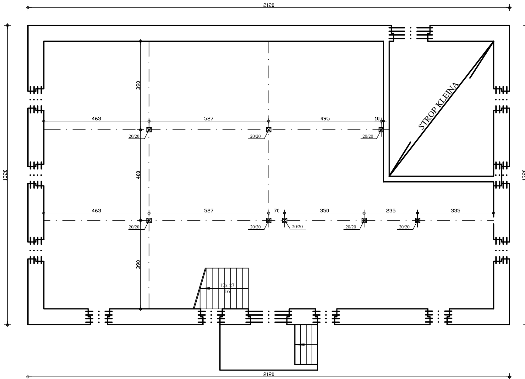
INWENTARYZACJA RZUTU KONSTRUKCJI PRZYZIEMIA skala 1:50
