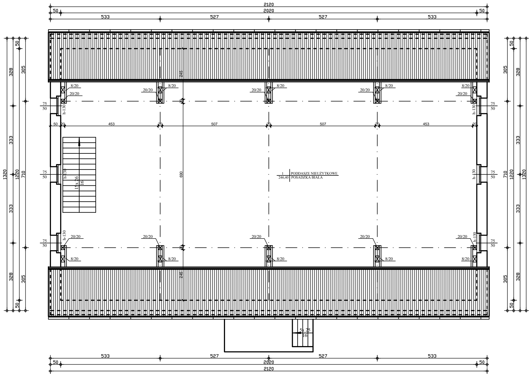
INWENTARYZACJA RZUT PODDASZA skala 1:50
