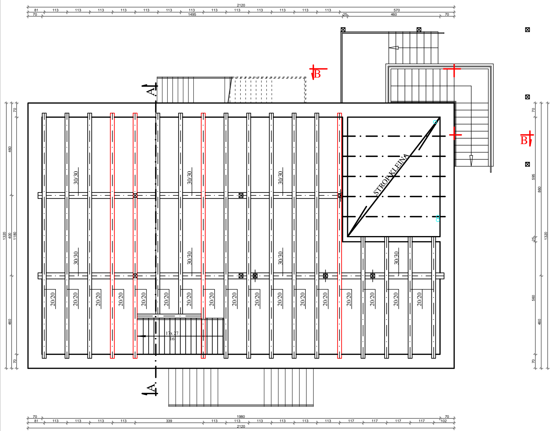
KONSTRUKCJA STROPU PRZYZIEMIA skala 1:50
