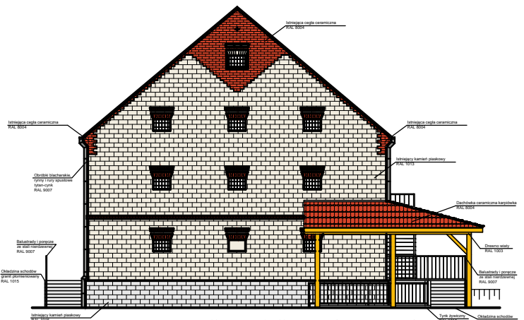
ELEWACJA BOCZNA /PRAWA/
