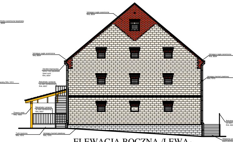
ELEWACJA BOCZNA /LEWA/
