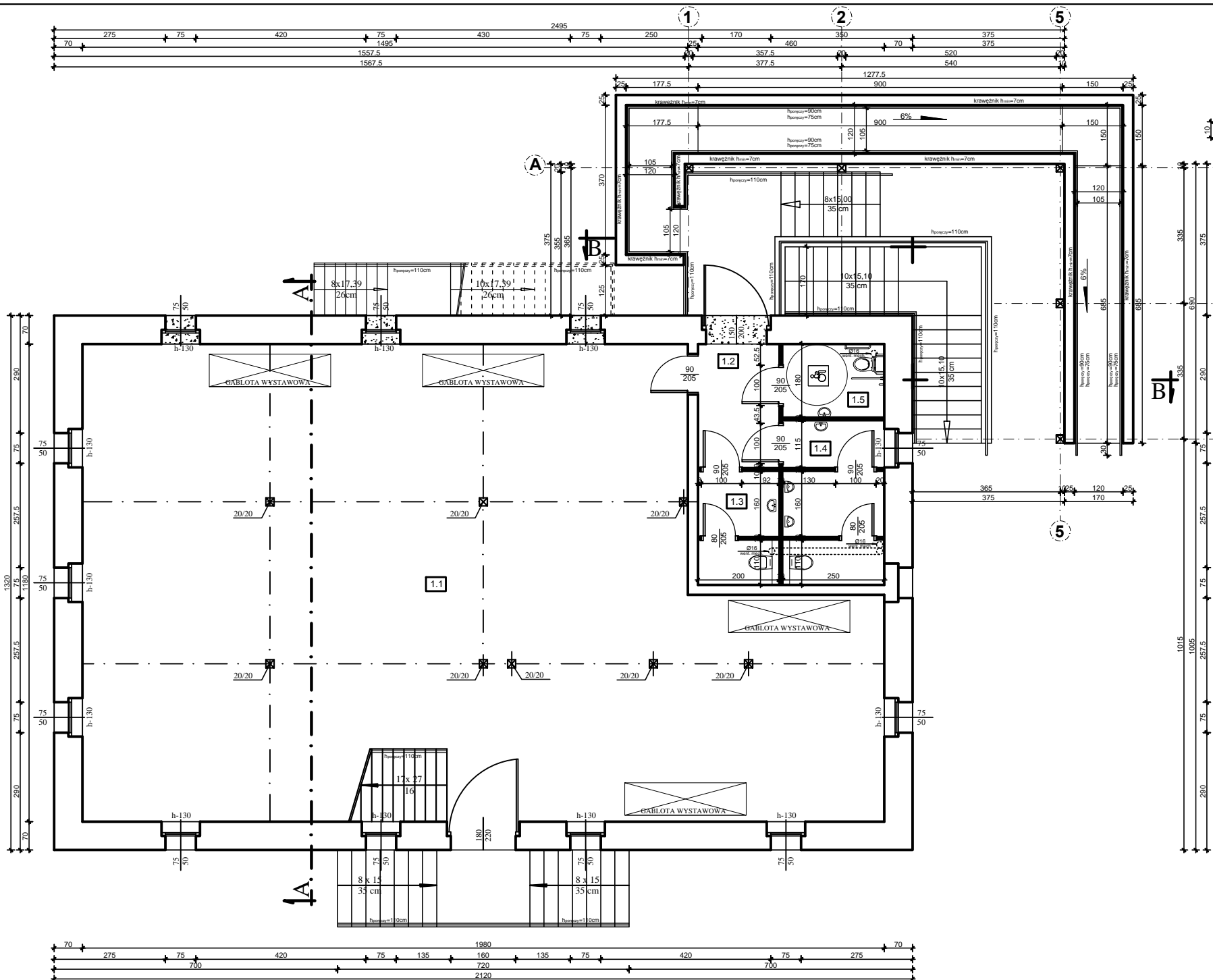
RZUT PRZYZIEMIA skala 1:50
