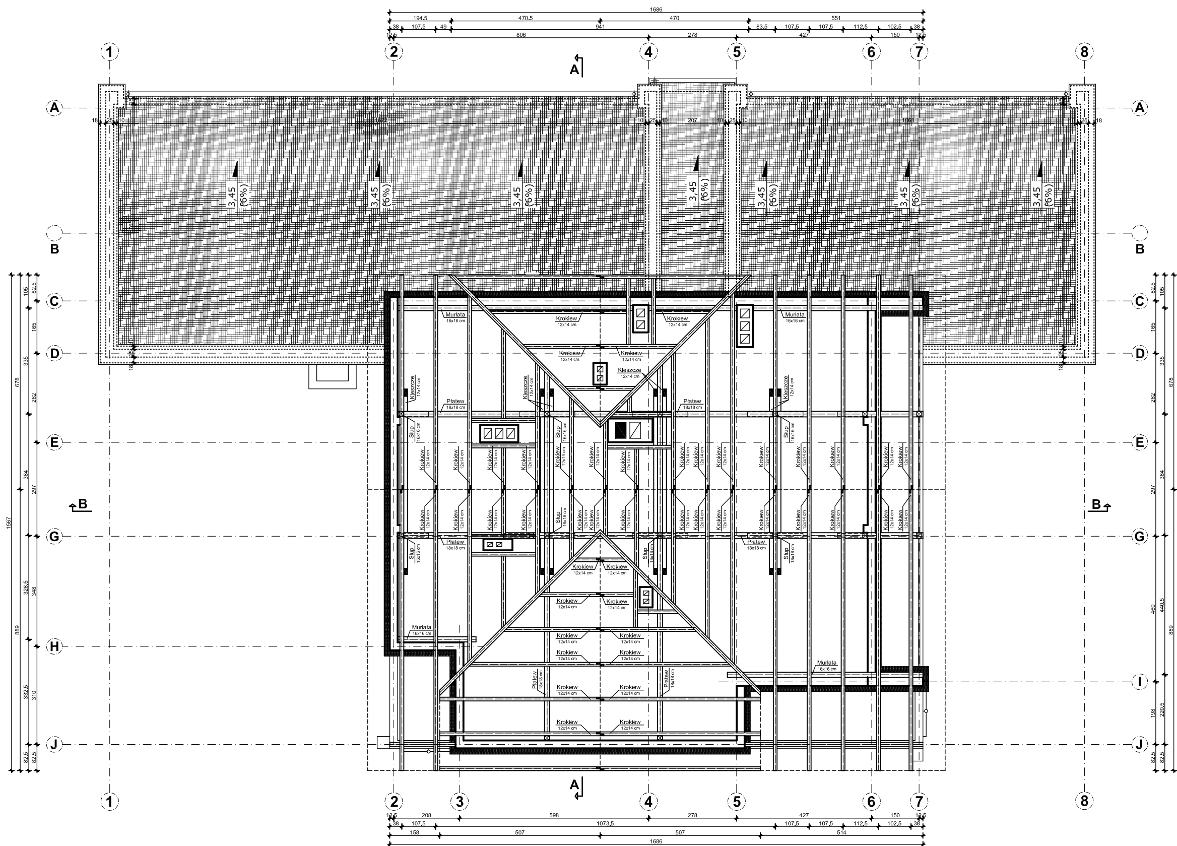
RZUT WIĘZBY DACHOWEJ skala 1:50
