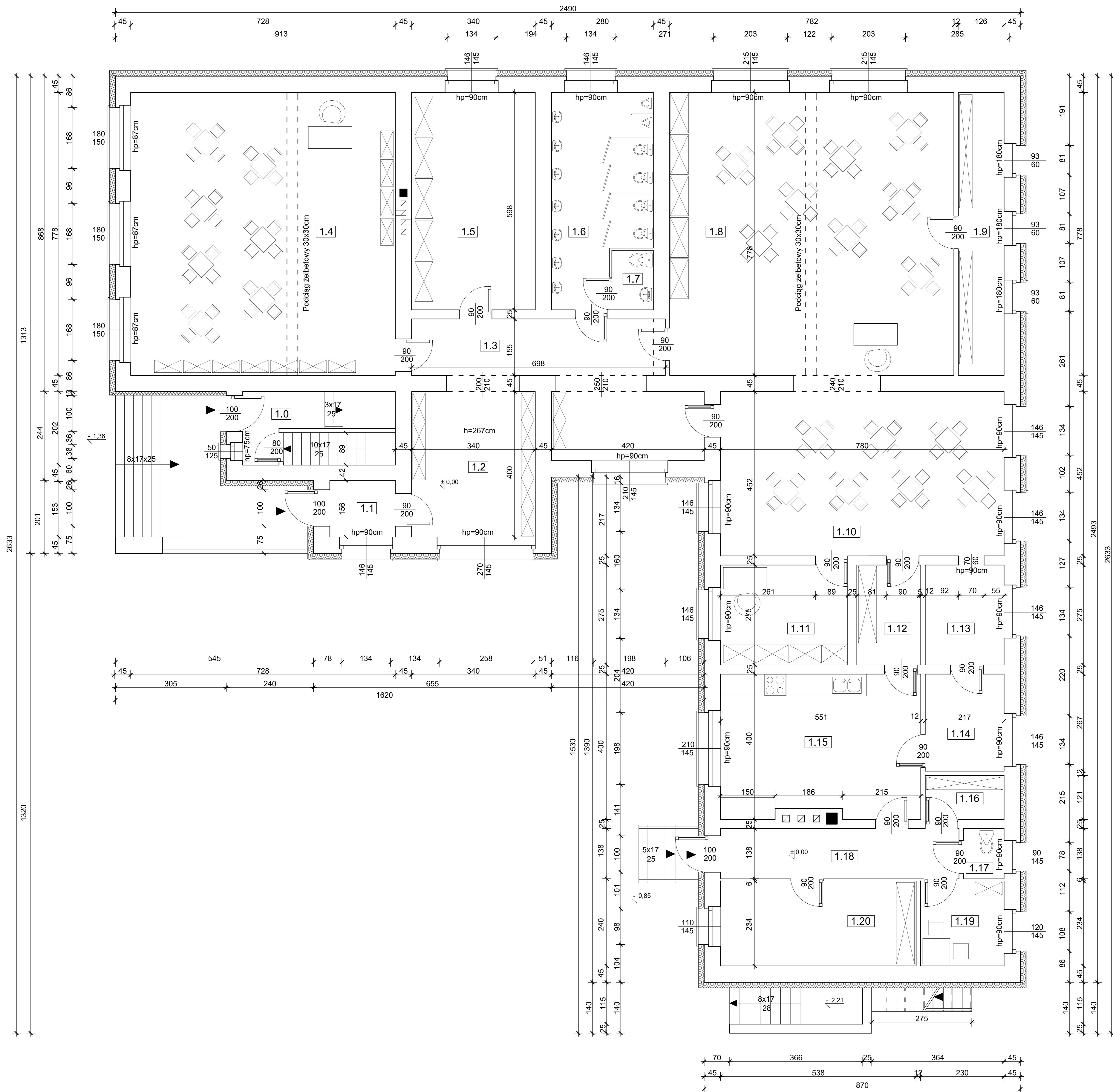
RZUT PARTERU - INWENTARYZACJA skala 1:50
