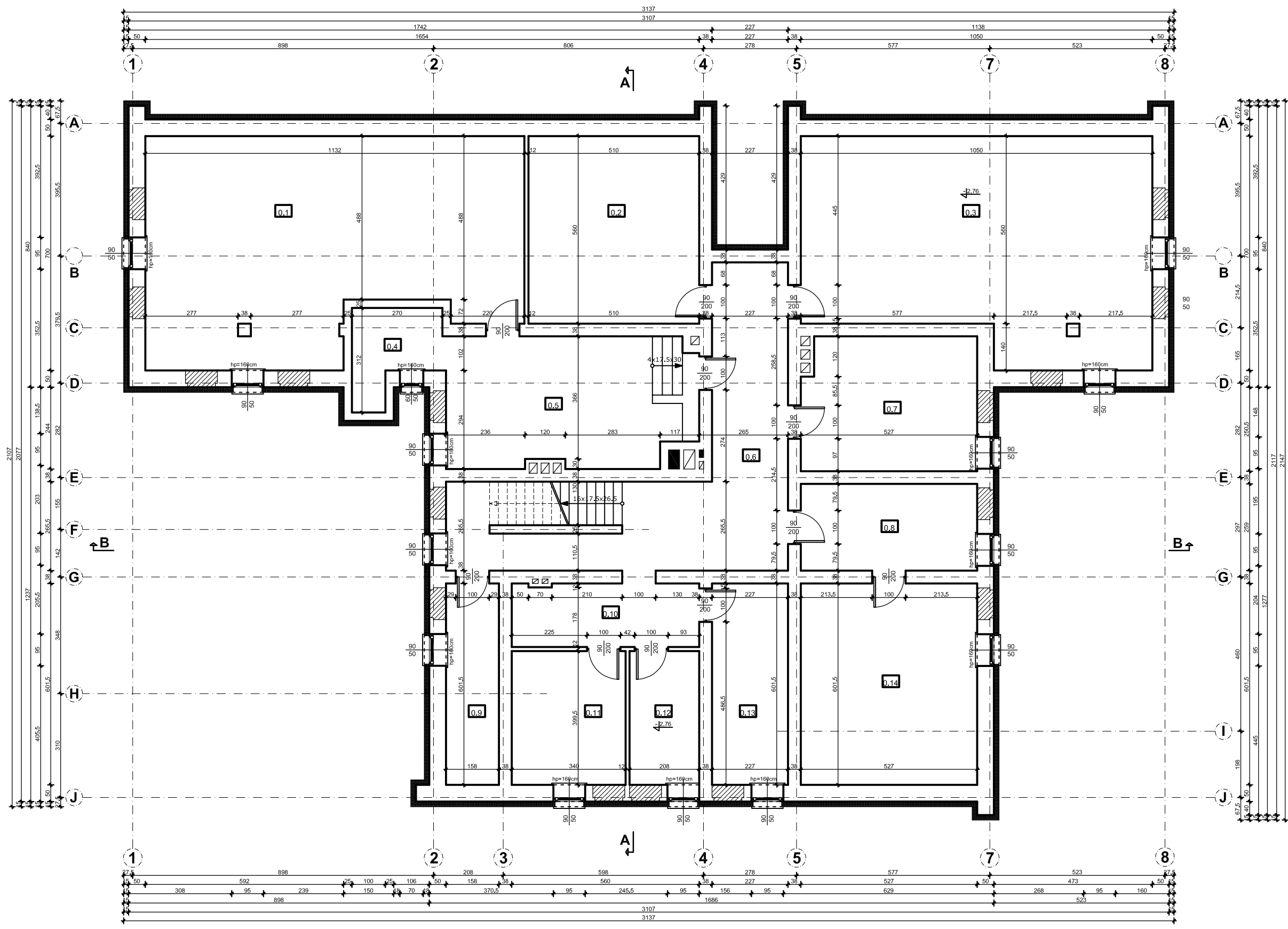
RZUT PIWNIC skala 1:50
