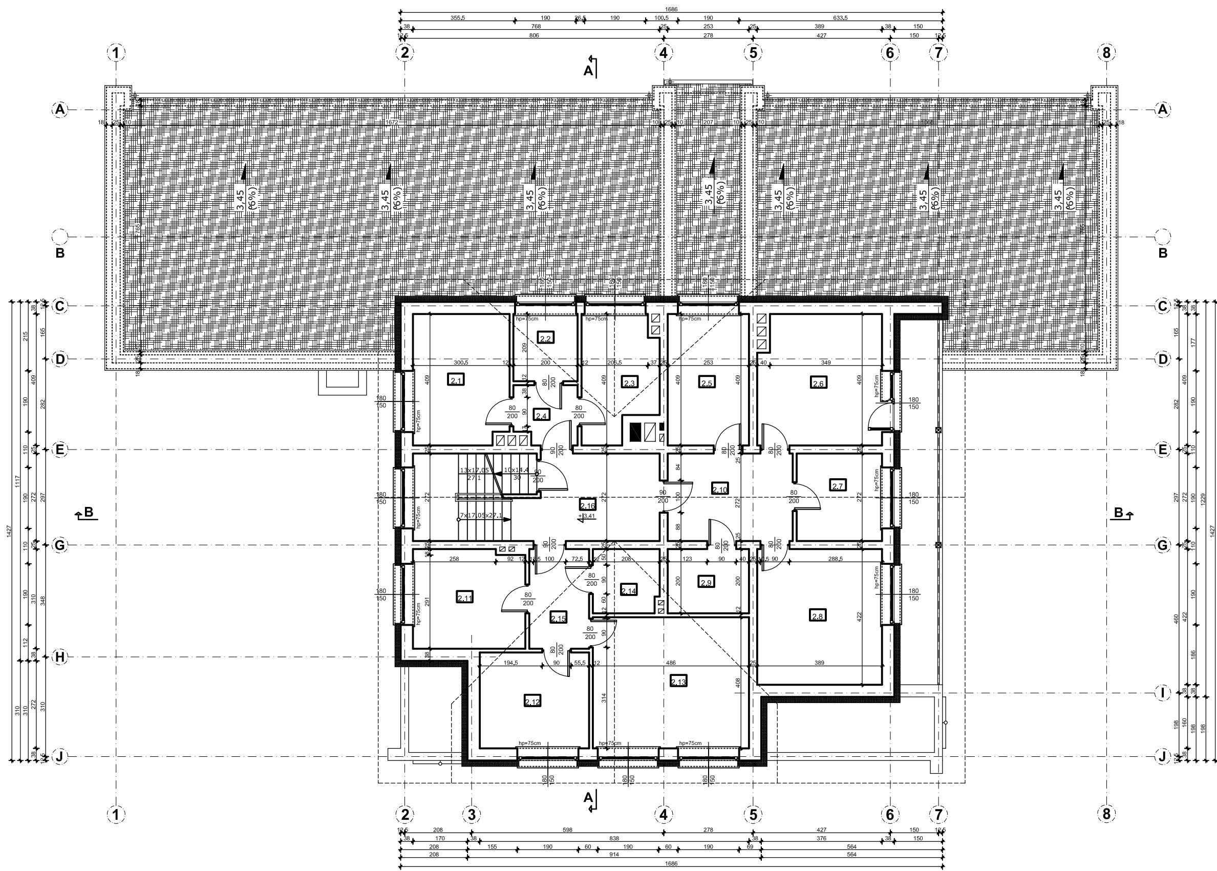
RZUT PIĘTRA skala 1:50
