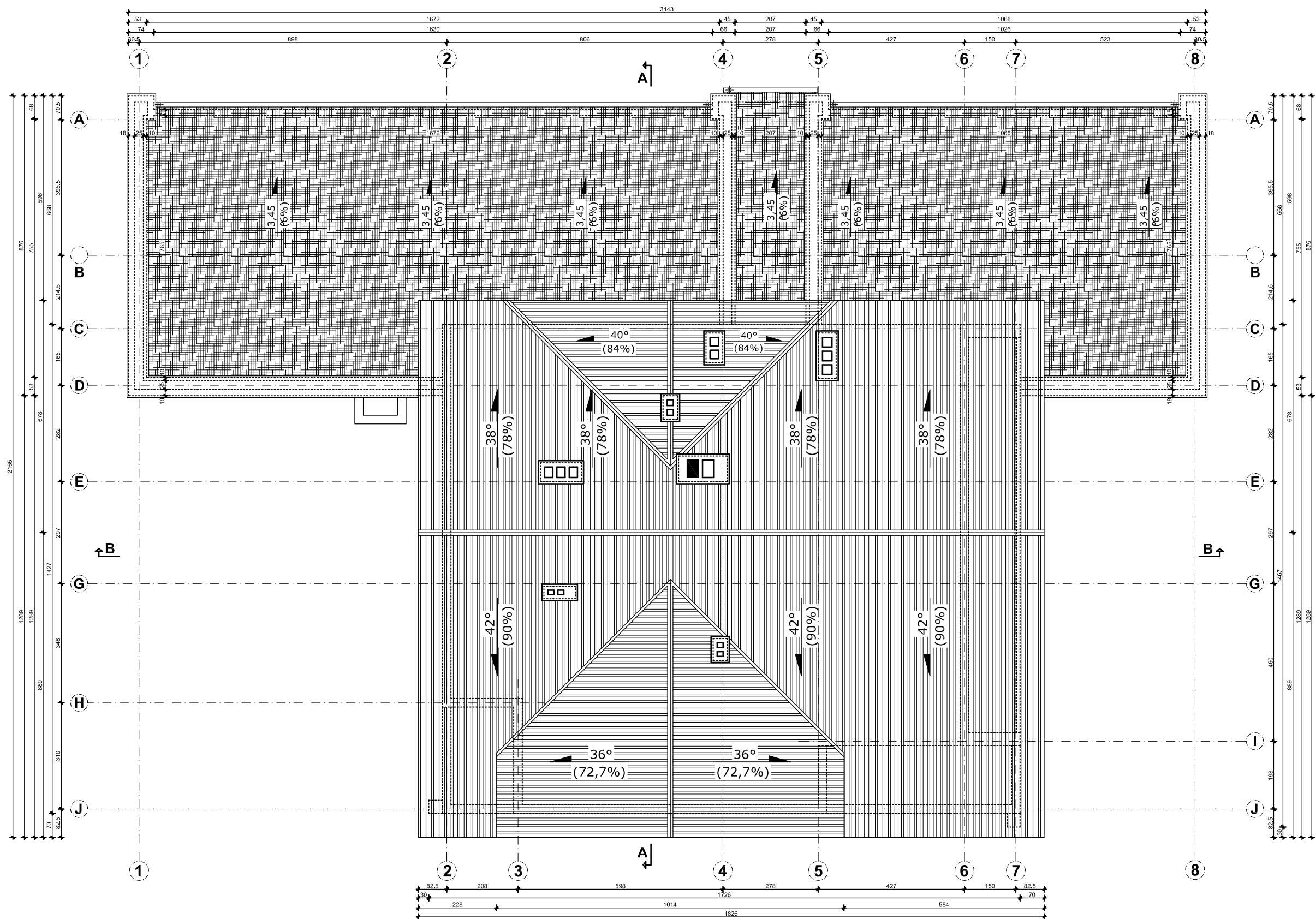
RZUT DACHU skala 1:50
