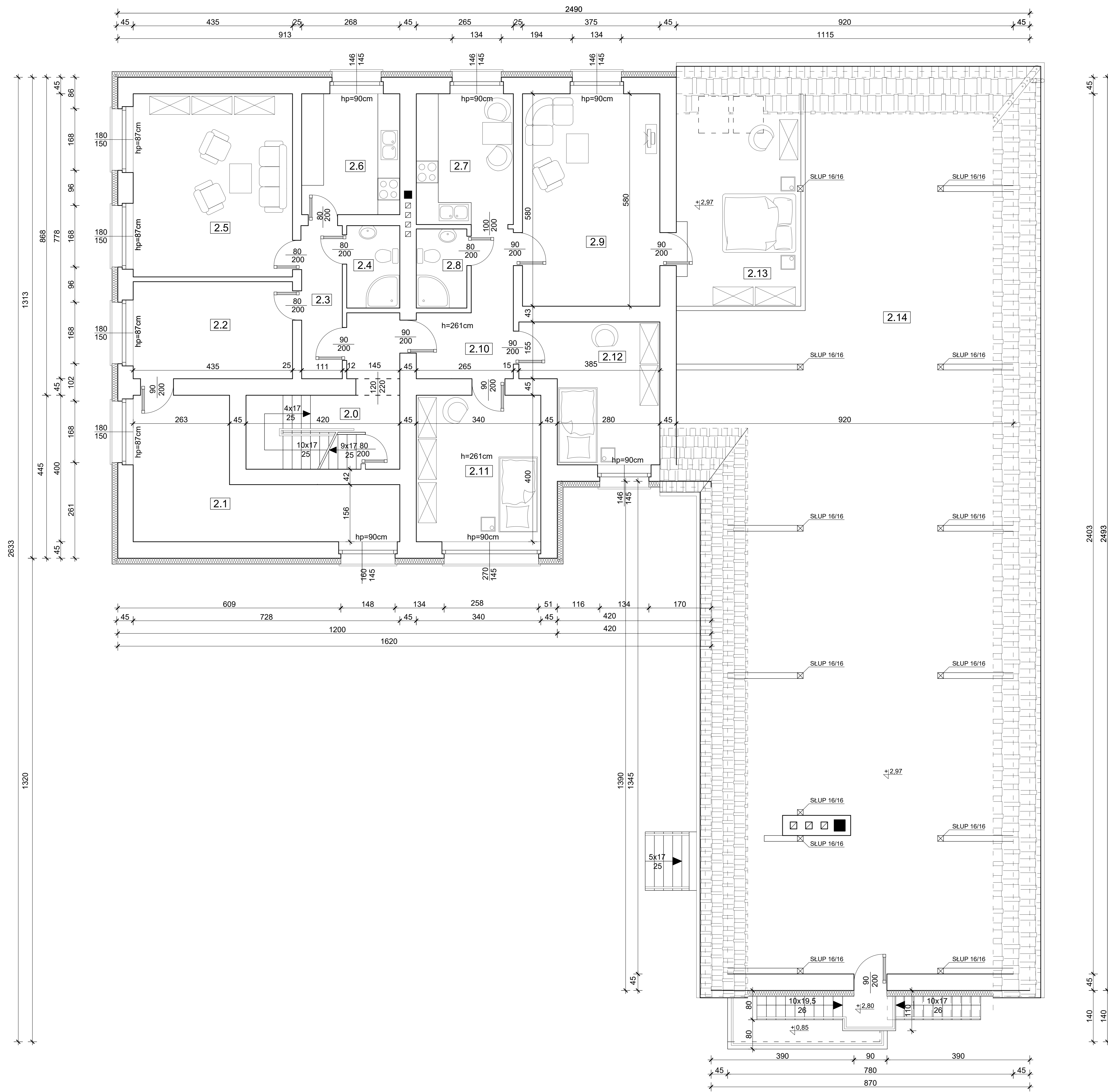
RZUT PIĘTRA - INWENTARYZACJA skala 1:50
