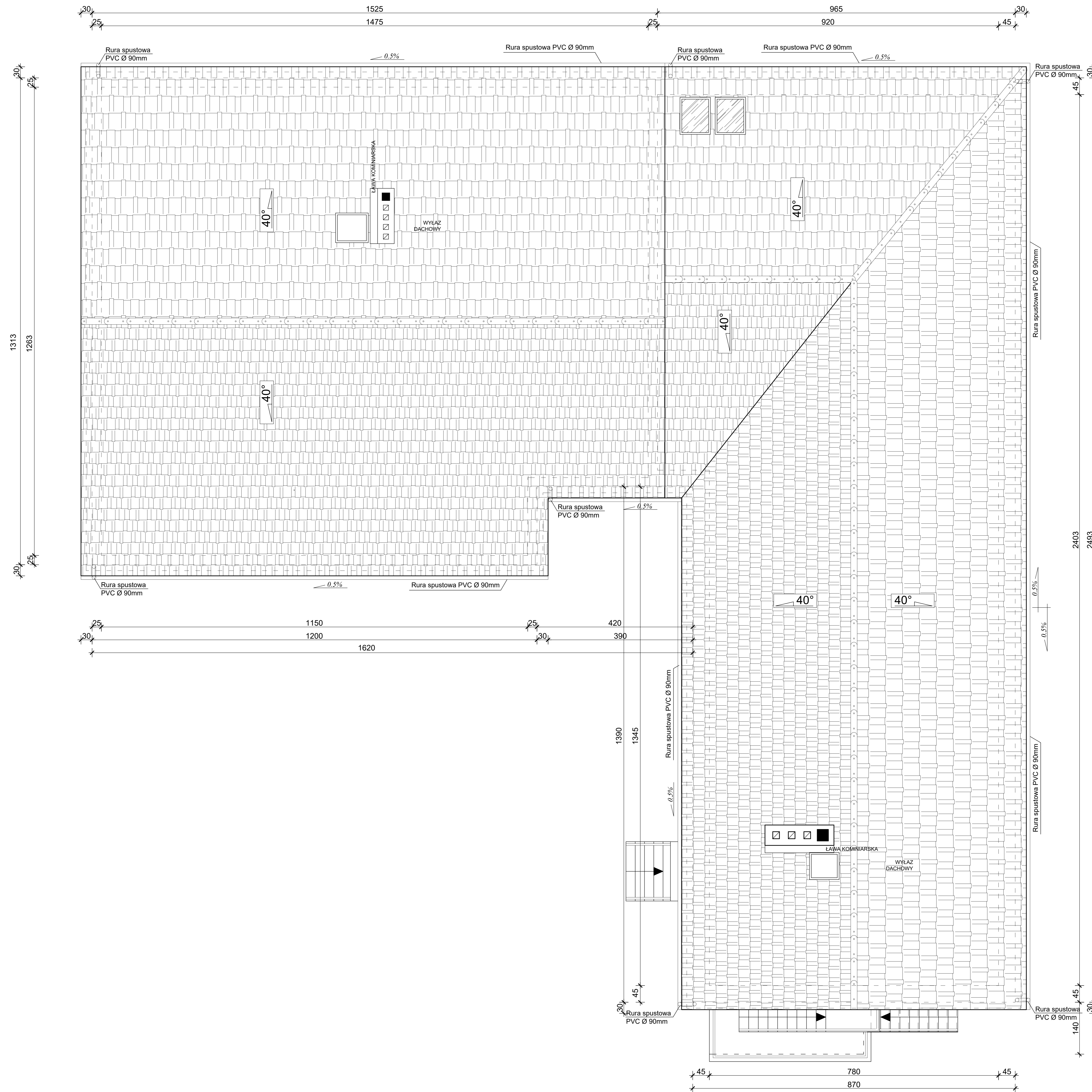
RZUT DACHU - INWENTARYZACJA skala 1:50
